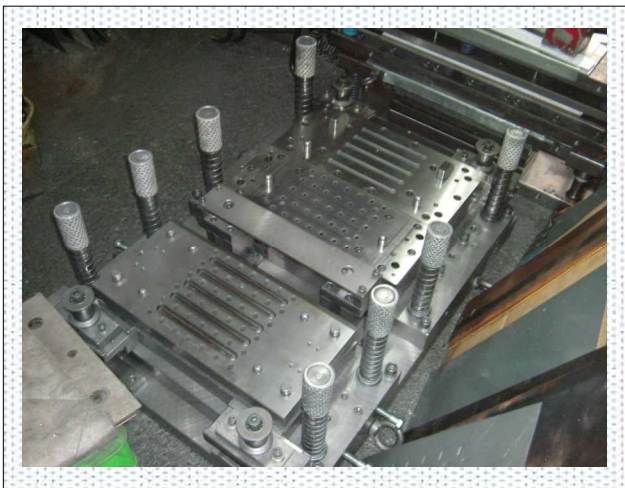
金型の写真
