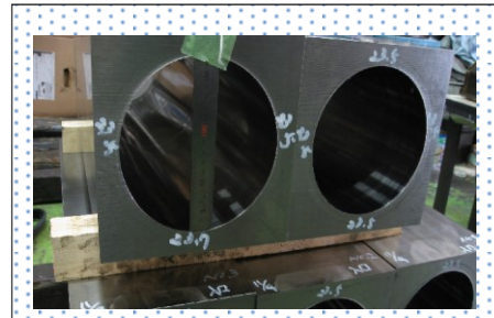
特殊材スーパーインバー φ168 210×210×680L 超制度の削孔
