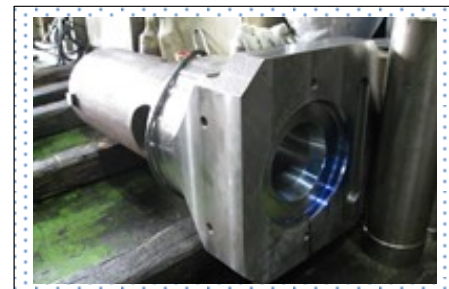
ダイキャストアルミ铸造 保安部品製造に必要なシリンダー
